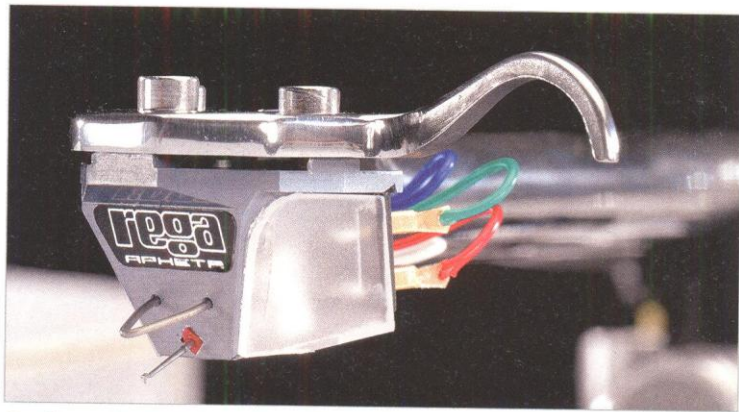
Das Rega-Apheta mit windschnittem Nadelschutz und Seitenspoilern
