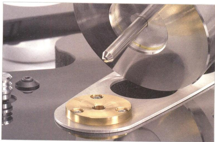
Klassisches Zero-Tolerance-Lager, links das hochpräzise Doppelpulley
